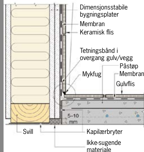
Prinsippkisse for overgang gulv/vegg (Tegningene er hentet fra Våtromsnormen)
